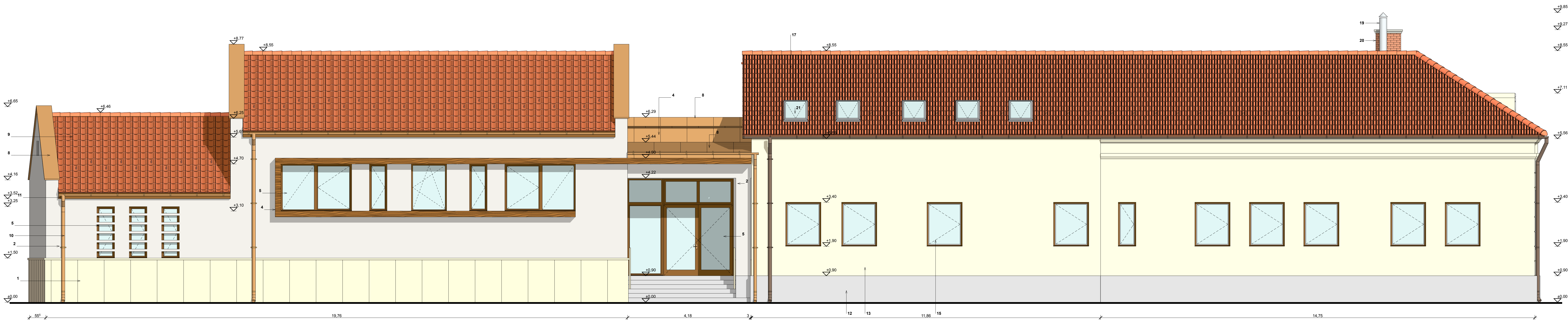
DÉLI HOMLOKZAT M 1:50
