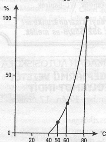
Vízkőképződés a melegvízhőmérséklet függvényében
