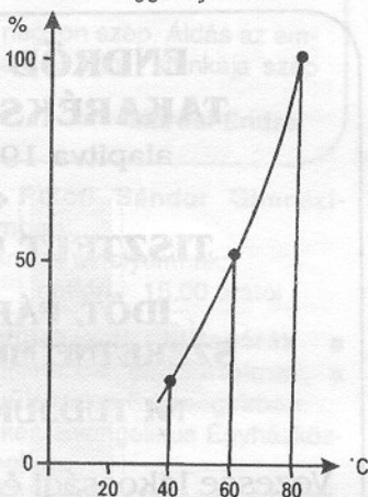
Hővesztesség a vízhőmérséklet függvényében
